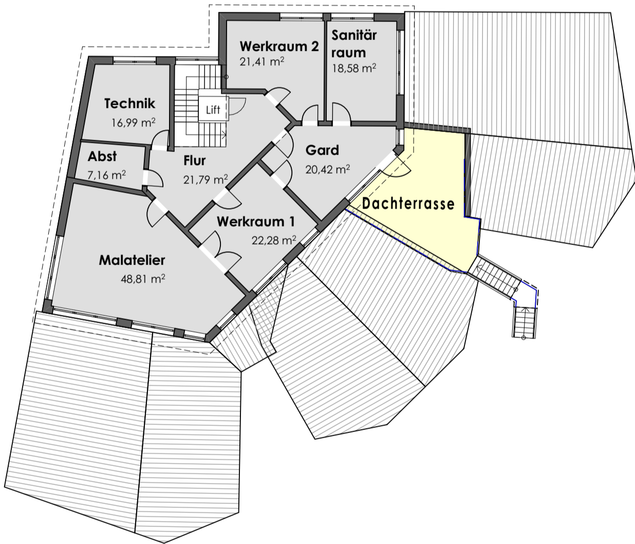
Grundriss OG bei 3 Gruppen
